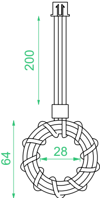
磁环 -150 A
